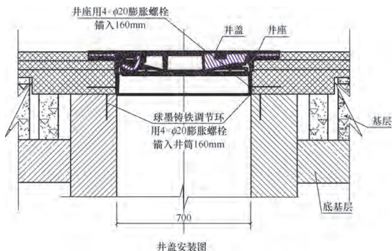
图 A.0.1 球墨铸铁宽边防沉降井盖安装图
